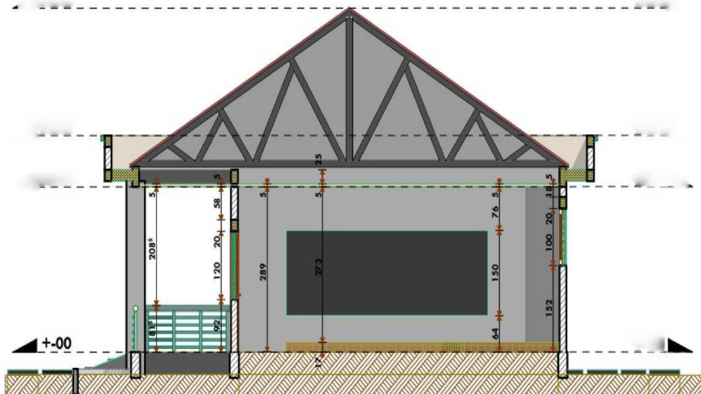
COUPE AA - SECTION AA
