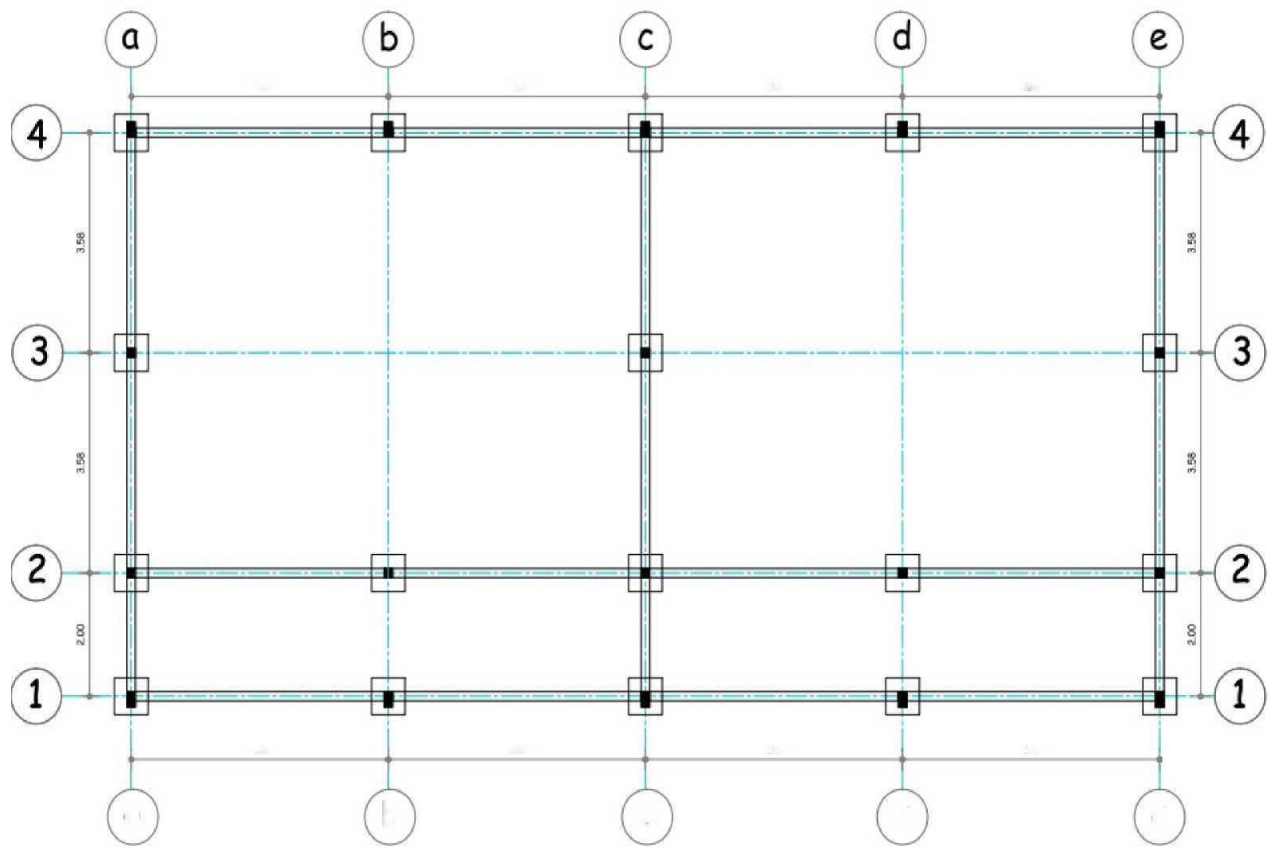
PLAN DE FONDATION - FOUNDATION PLAN
